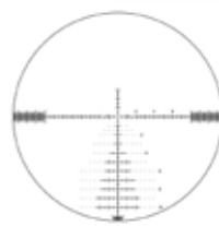
G4P Precision Absehen in 1. Bildebene
